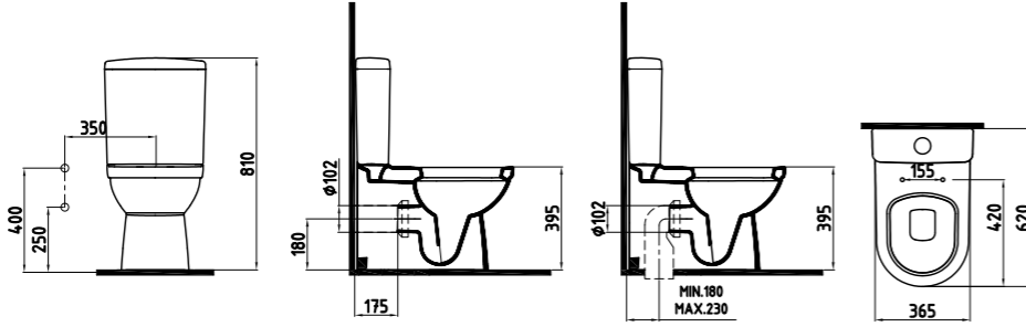
DORADO DUVARA SIFIR KLOZET 620 mm CPKD06201VS1W5QAO Taharet borusu, 90° körüklü kada, çekirtilmeli montaj seti, delik iptal tapası, spiral hortum geçme adaptörü ve spiral hortum dahildir. Duroplast klozet kapağı ve iç takım dahil değildir.
