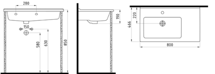
KONSOLLU SAĞDAN ETAJERLİ LAVABO NPLK080B2FD1W5QA0 810x470 mm
