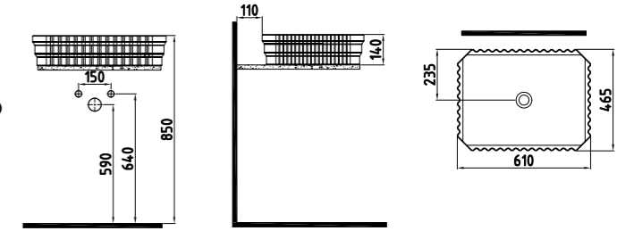
GÖVDE ÜSTÜ LAVABO BATARYA DELİKSİZ SHLG06101FD0W5QA0 610x465 mm
