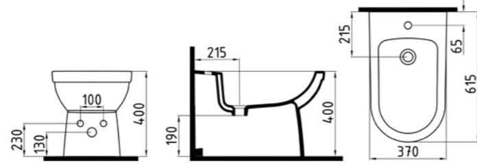
DORADO YERDEN BİDE 620 mm CPBY06201VD1W5QAO Tek delikli.
