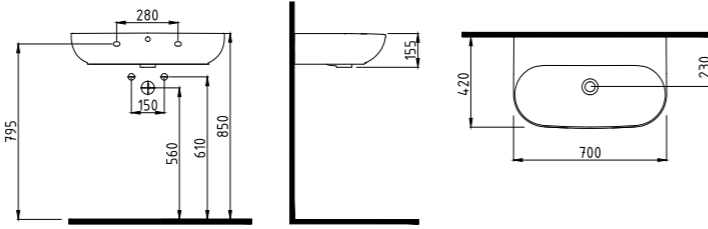
GÖVDE ÜSTÜ LAVABO BATARYA DELİKLİ MDLS07001FD1W5QA0 700x420 mm
